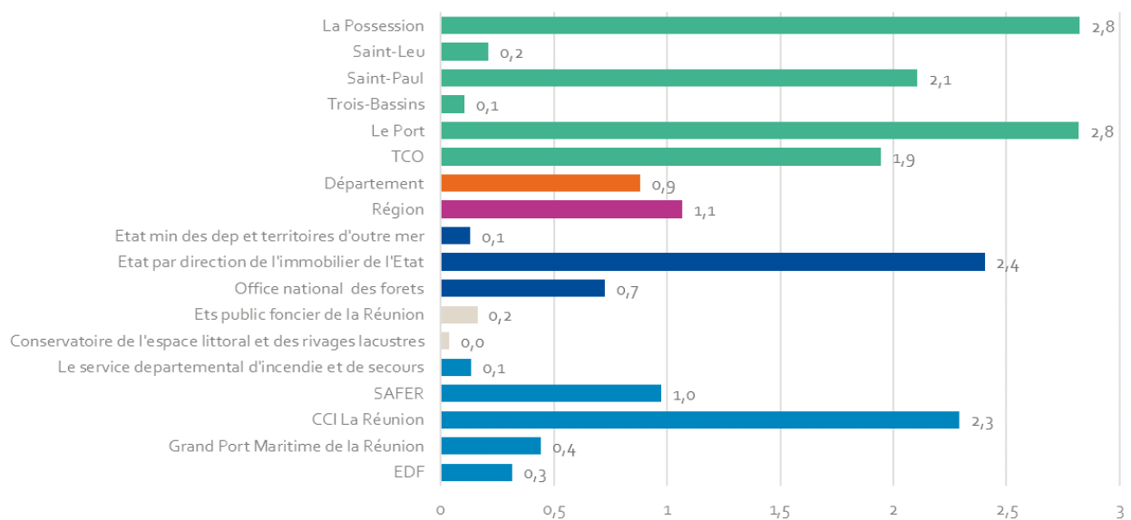
Figure 44 : Répartition de la puissance installable par propriétaire (source : cadastre solaire)
