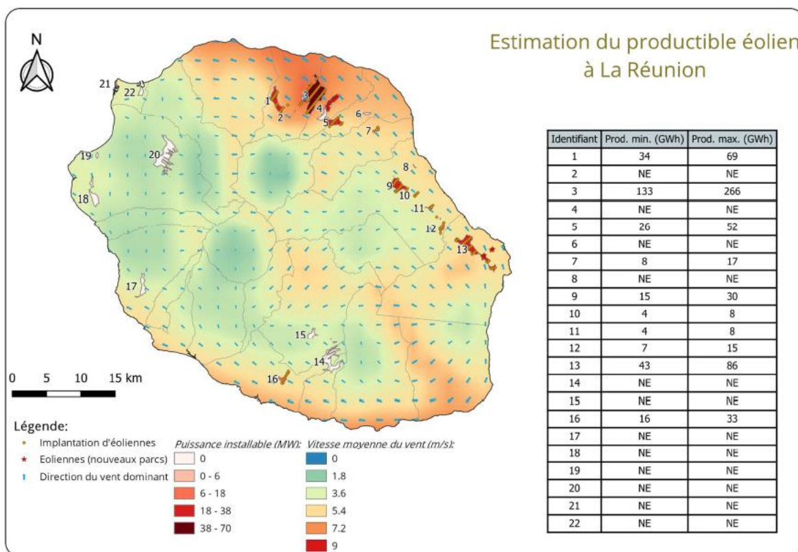
Figure 46: Estimation du productible éolien à La Réunion (Source : Schéma Régional éolien de La Réunion 2022 – version provisoire)
