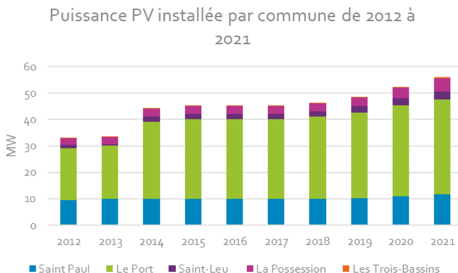
Figure 38: Cumul des puissances PV par commune sur la période 2012-2021 (connecté au réseau) (Sources : OER, EDF)
