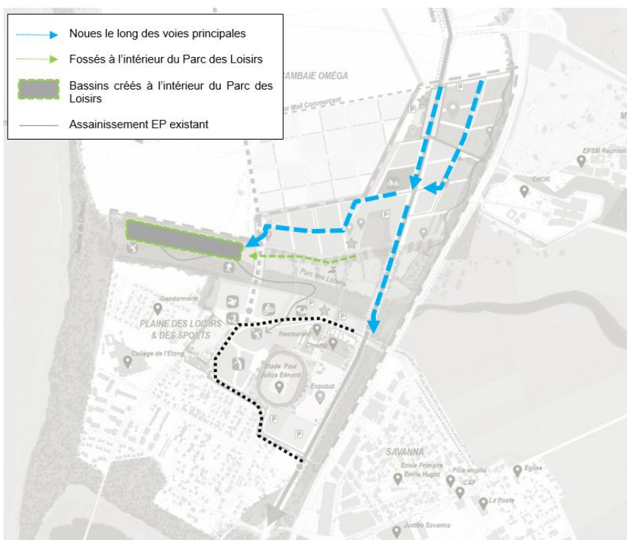
Fig. 39. Gestion des eaux pluviales du projet Cambaie Oméga
