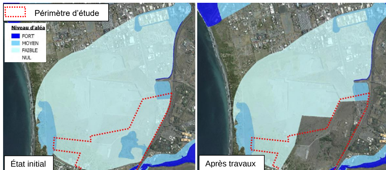
Fig. 38. Zonage d'inondation avant travaux de dérivation des eaux (à gauche) et après travaux (à droite)
