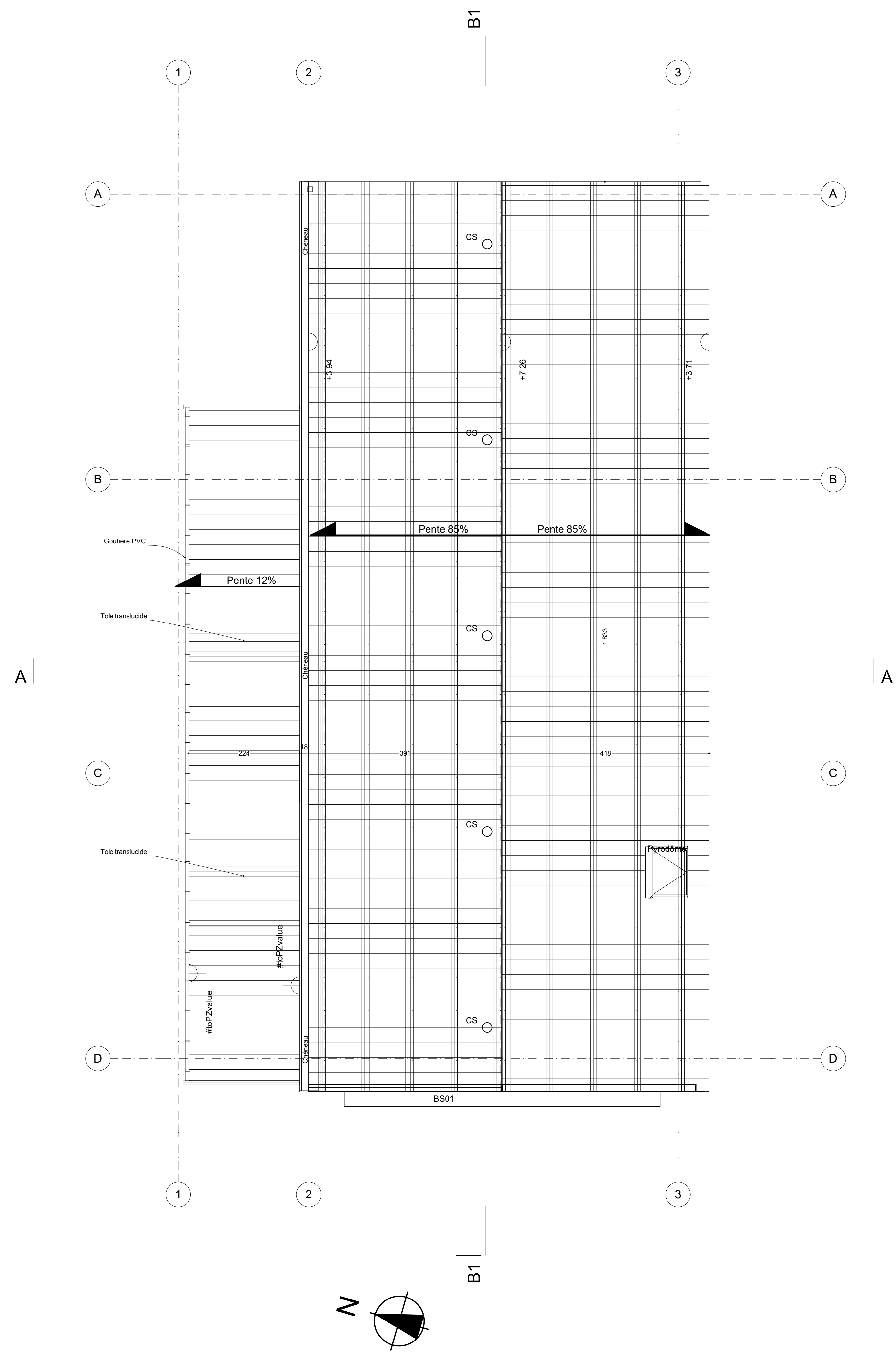
Toiture
