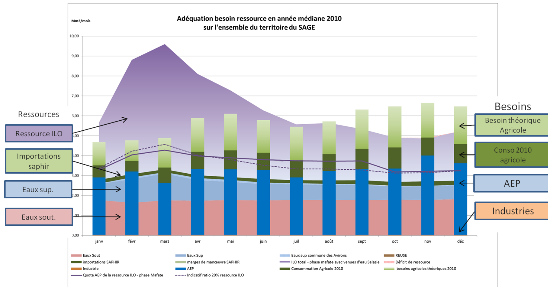
Figure 5: Analyse Ressource Besoin en année médiane 2010 sur le territoire du SAGE
